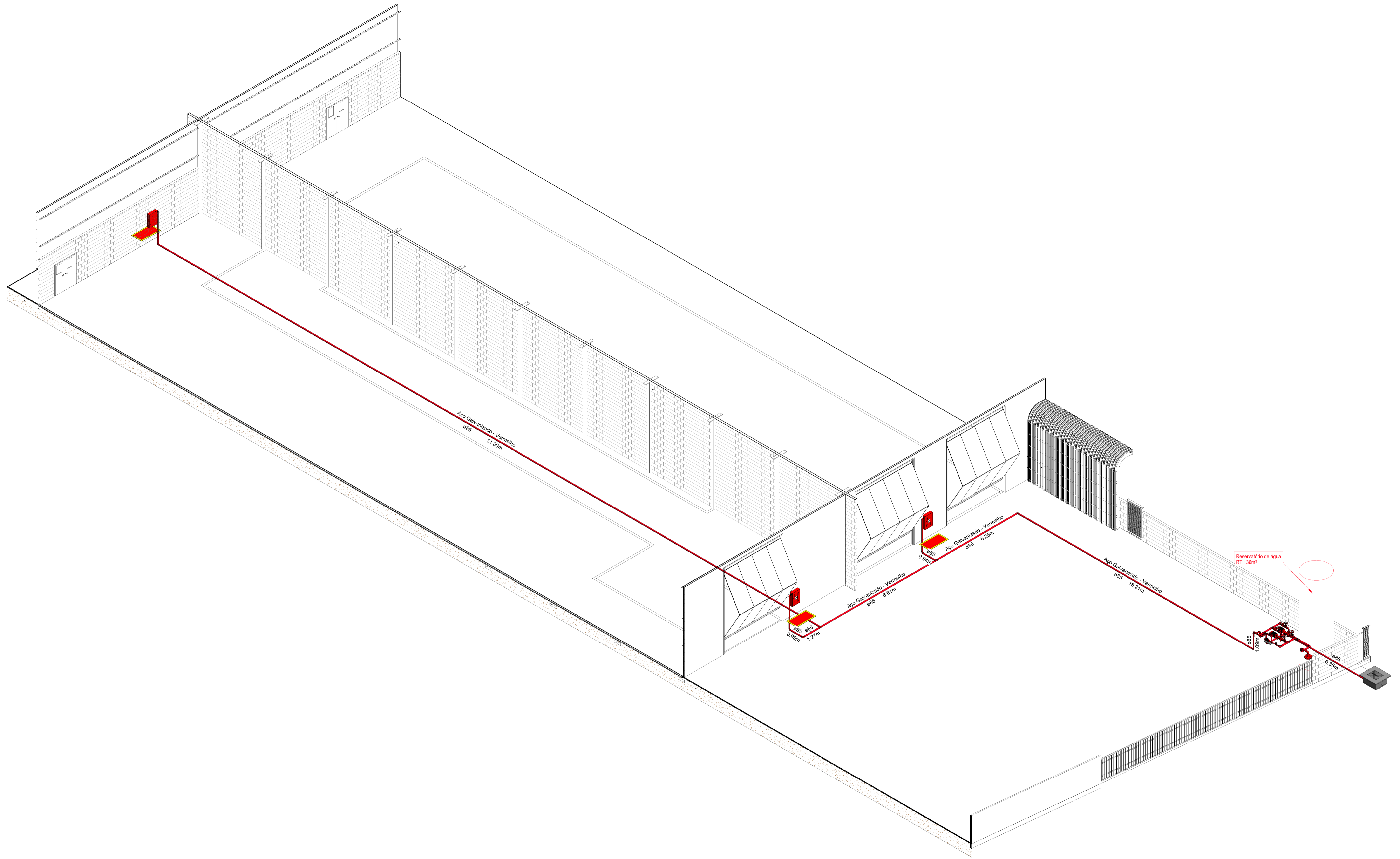
1 Hidrantes-Vista isométrica
